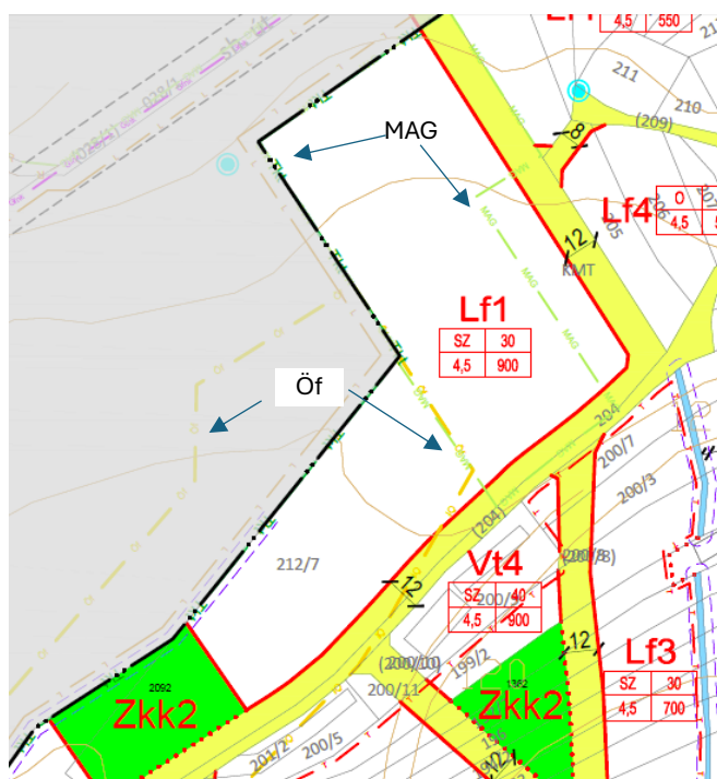
Ábra 1: Örvényes Község Önkormányzata Képviselő-testületének 1/2017.(III.13.) önkormányzati rendelete a helyi építési szabályzatról - 1. melléklet (SZT-1)
