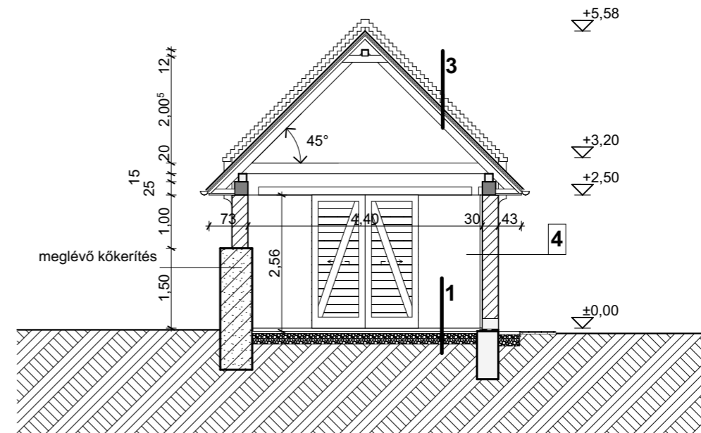
B-B metszet
