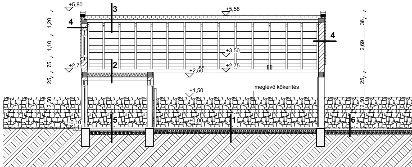
A-A metszet
