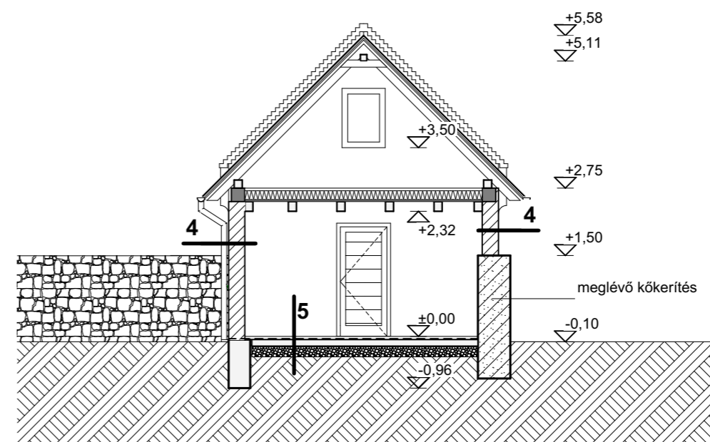
C-C metszet
